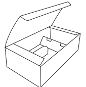
Unica 2 Bott. 340x180x95 Art. 137721S 3 Bott. 340x270x95 Art. 137722S
